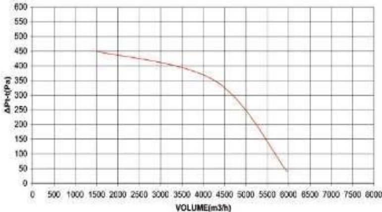
Φ250-1.5HP-1450RPM
